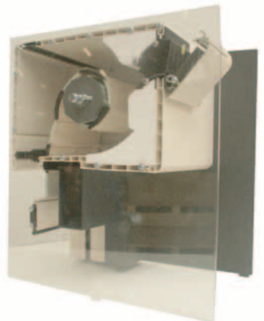
DÉCOUPE ROLVENT® VOLET
